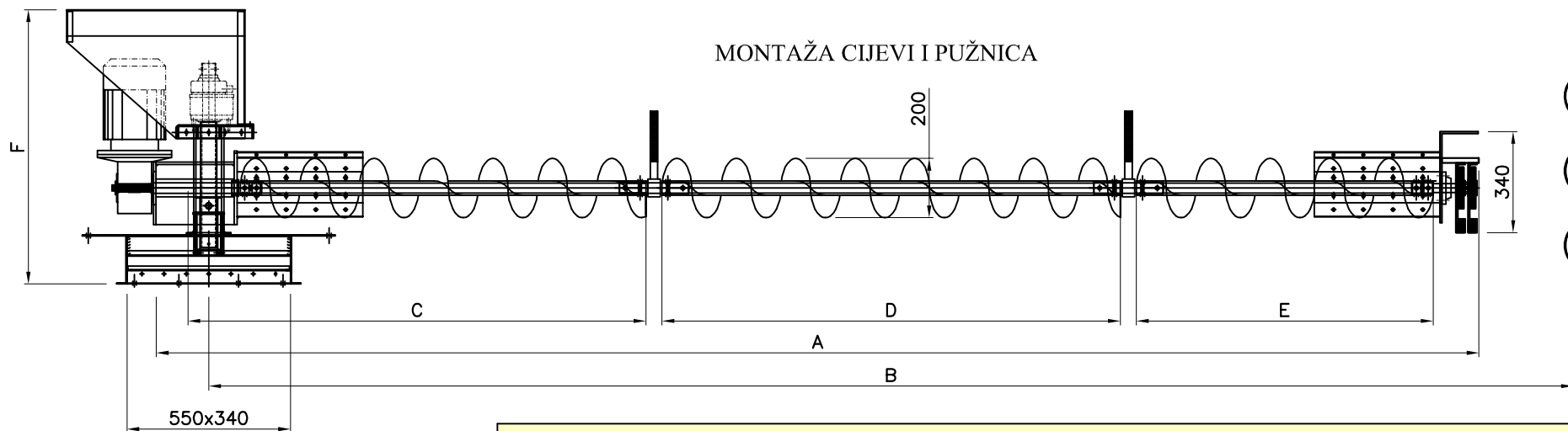
MONTAŽA POKLOPACA
